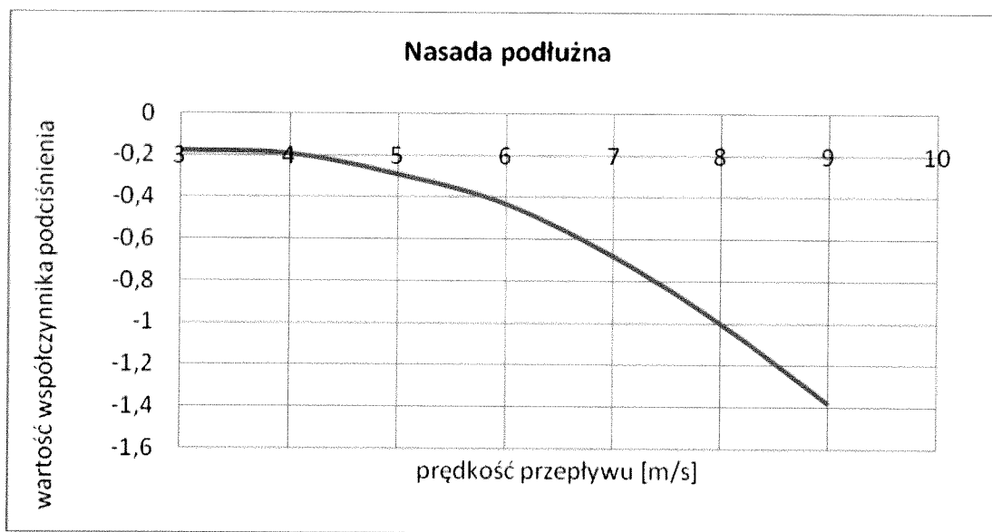
Rys. 3 Współczynnik podciśnienia nasady kominowej podłużnej typ KJ40 przy zerowym przepływie.
