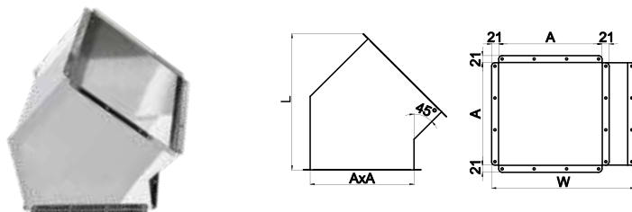
Chute elbow 45°
