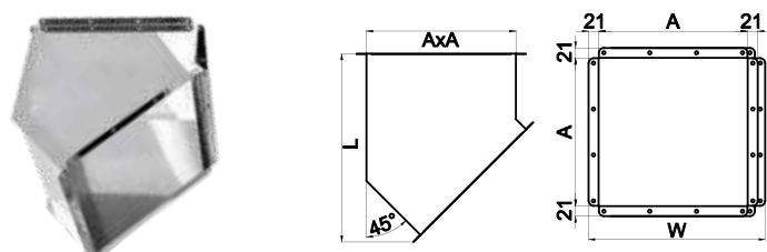
Chute end 45°
